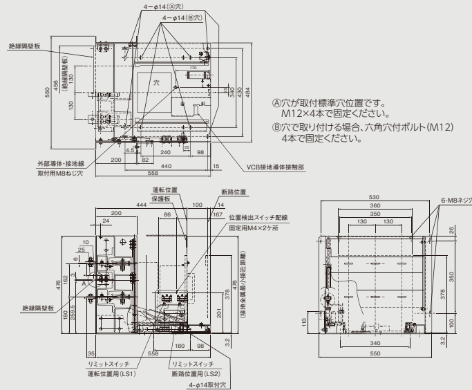
■遮断器固定枠外形寸法図
