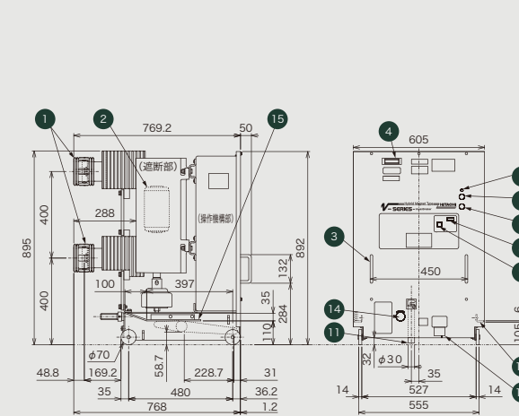
■遮断器外形寸法図
