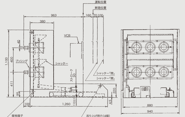
■遮断器固定枠外形寸法図
