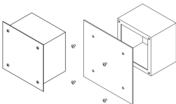
張り出しふた
