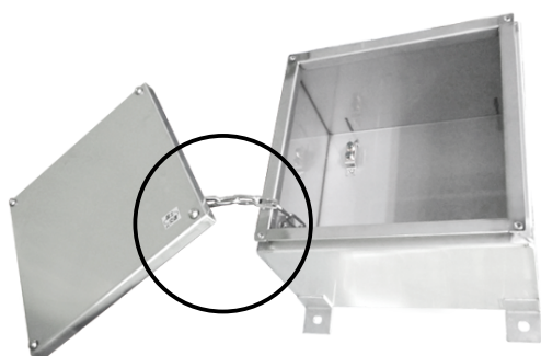
ふた落下防止チェーン取付
