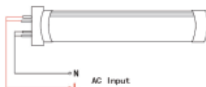
電源直結工事：結線図(側面)
