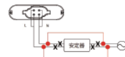
電源直結工事：結線図(正面)
