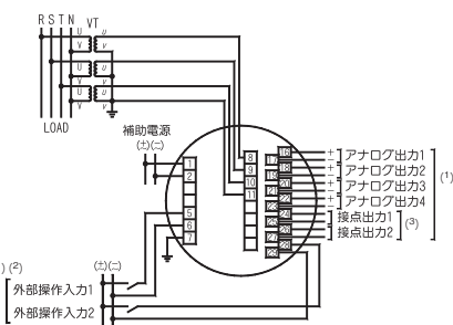
図-23 電圧入力 三相4線(3VT)
