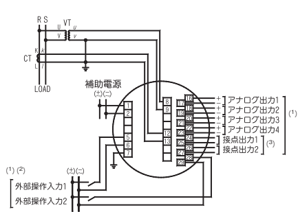
図-1 単相2線
