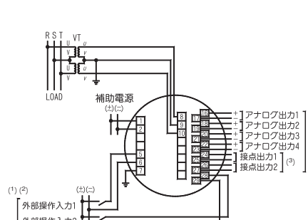
図-12 三相3線
