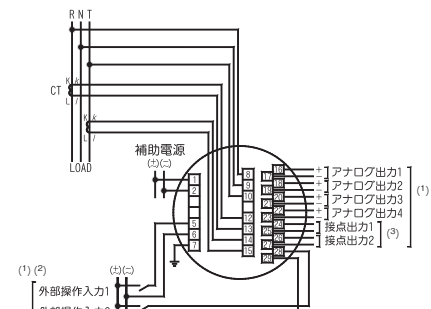
図-2 単相3線
