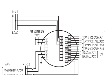
図-11 単相3線
