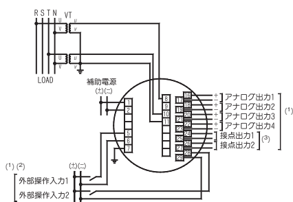
図-22 電圧入力 三相4線(2VT)
