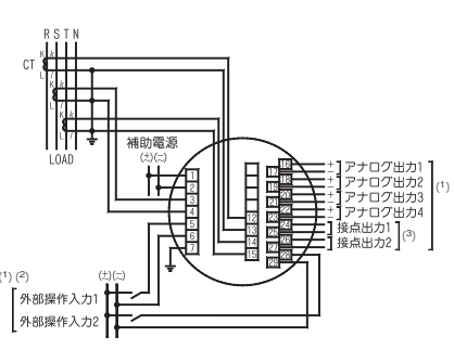
図-21 三相4線(3CT)
