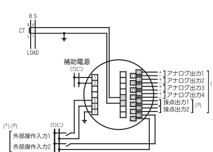
図-5 単相2線
