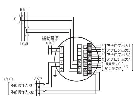
図-6 単相3線
