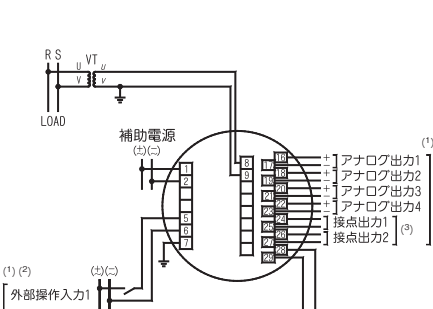
図-10 単相2線
