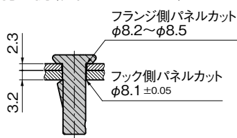
取付け例 (板厚2.3mm+3.2mm)
