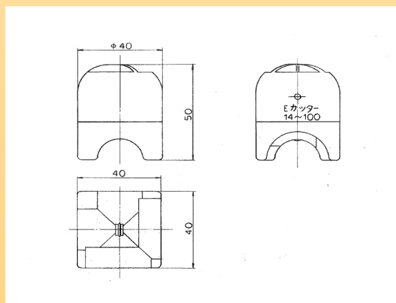
Eカッター(小)図面
