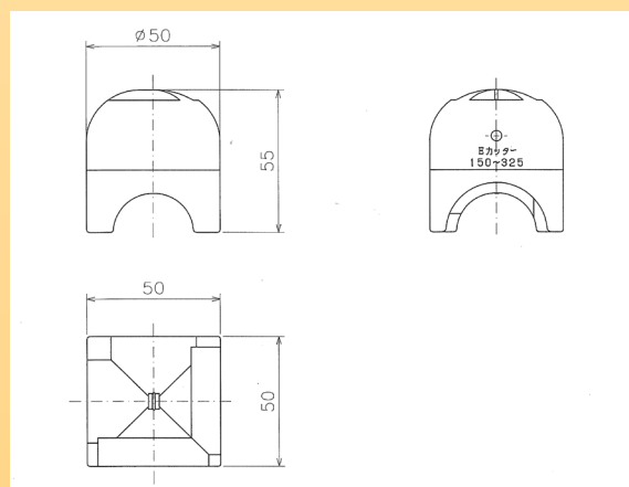
Eカッター(大)図面
