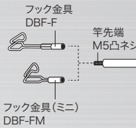
フック金具 DBF-F
