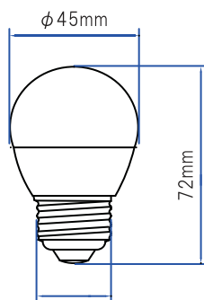
製品寸法図
