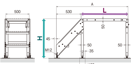
片階段 キット
