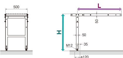
延長 キット
