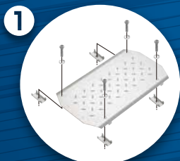
連結金具
