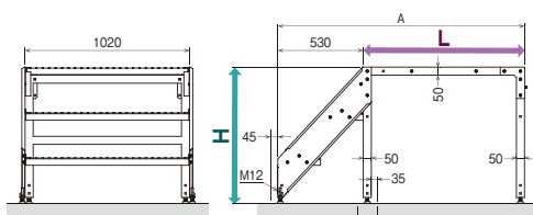
片階段 キット
