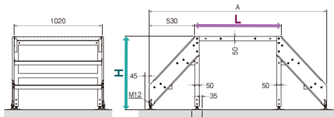
両階段 キット
