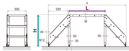
両階段 キット
