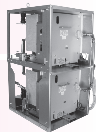
VSS-6D4E 分割引出形 VSS-6D4E Breakup drawout type
