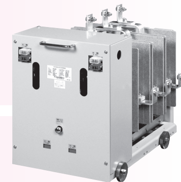
VSS-6H4 固定形 VSS-6H4 Fixed type
