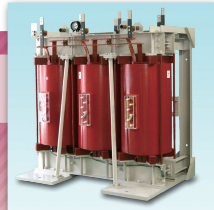
▲浮体式洋上風力発電用昇圧変圧器
