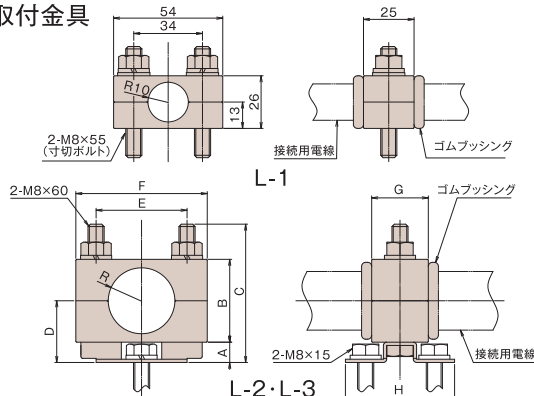
電線取付金具
