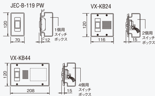
■寸法図(mm)
