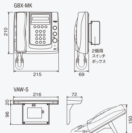
■寸法図(mm)
