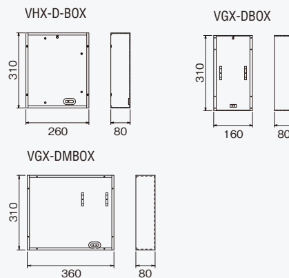
■寸法図(mm)
