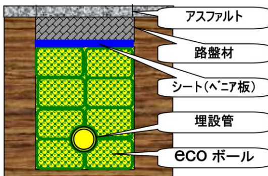
■ecoボール施工イメージ
