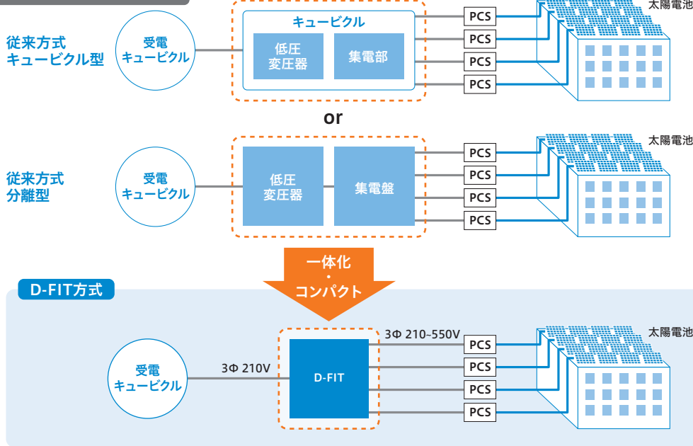
従来方式との比較(250kVAの例)
