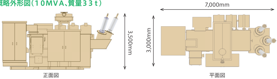
【参考】概略外形図(10MVA、質量33t)
