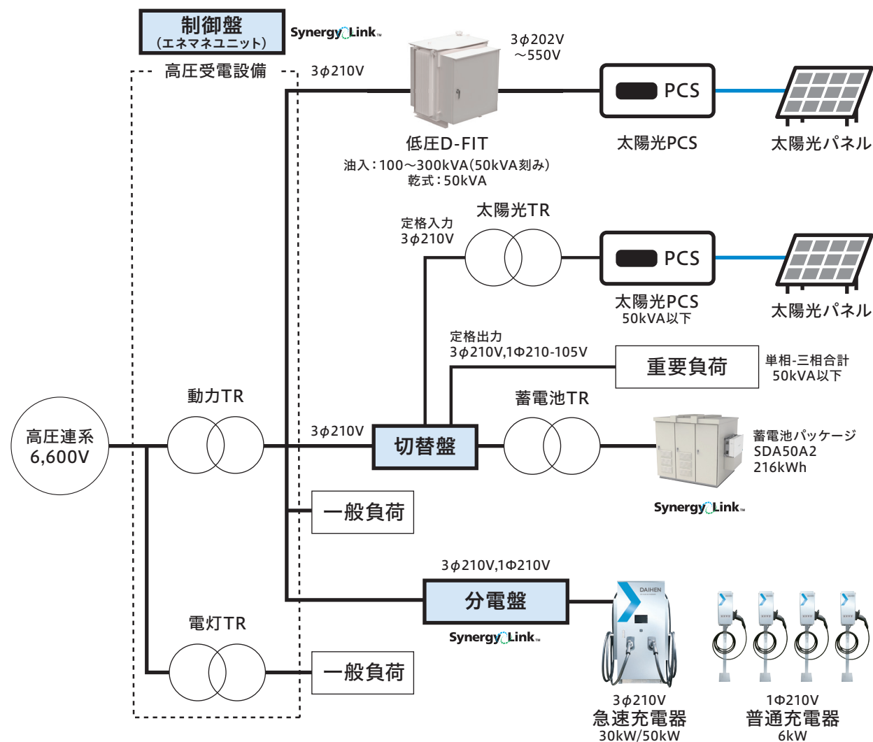
太陽光設備・蓄電池・EV用充電器を導入する場合
