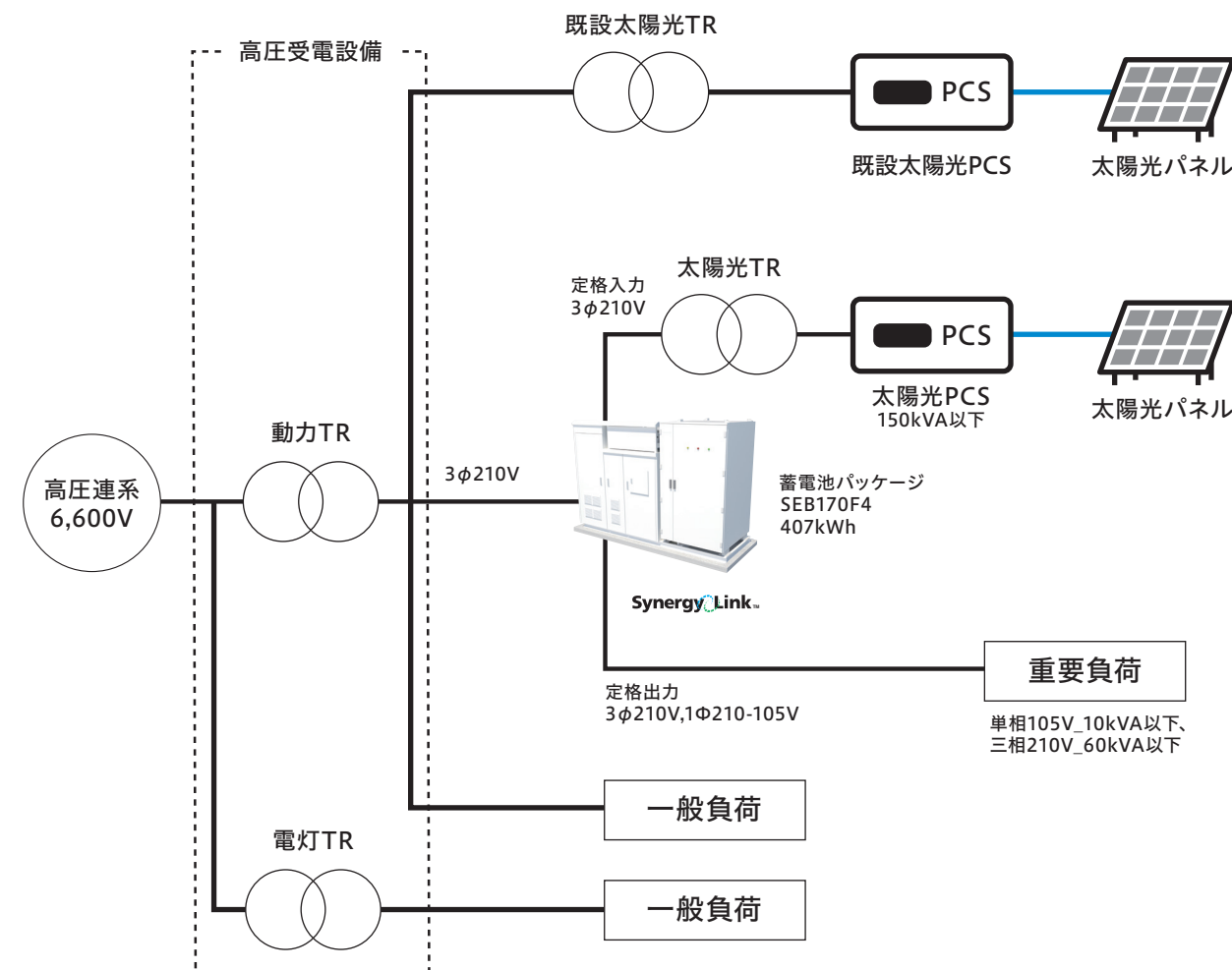
既設の太陽光設備に蓄電池を導入する場合
