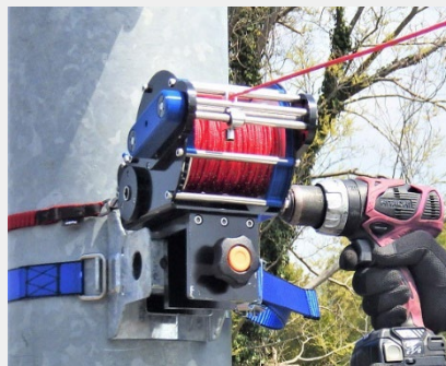
小型ロープ巻取機
