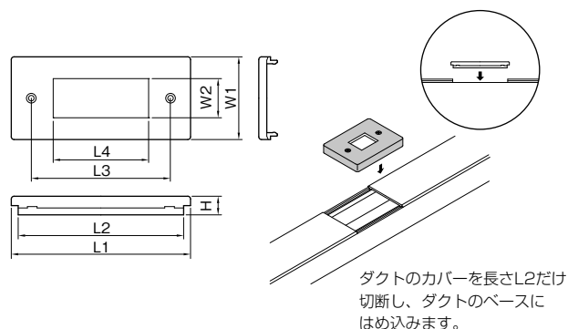
LANモジュージャック使用例
