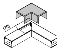
45°カット接続時施工例
