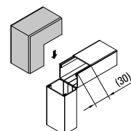
突当て接続時施工例
