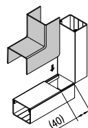
突当て接続時施工例1
