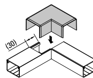
突当て接続時施工例
