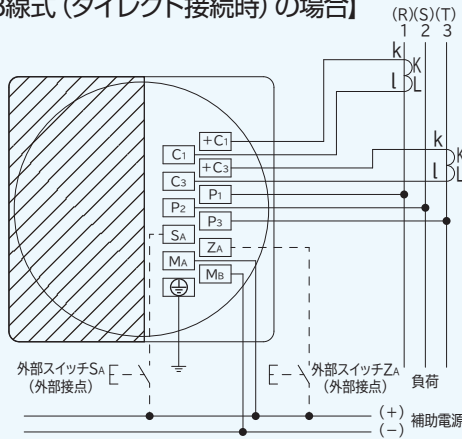
【三相3線式 (ダイレクト接続時) の場合】
