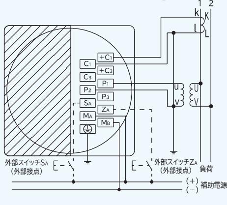
【単相2線式 (VT使用時) の場合】
